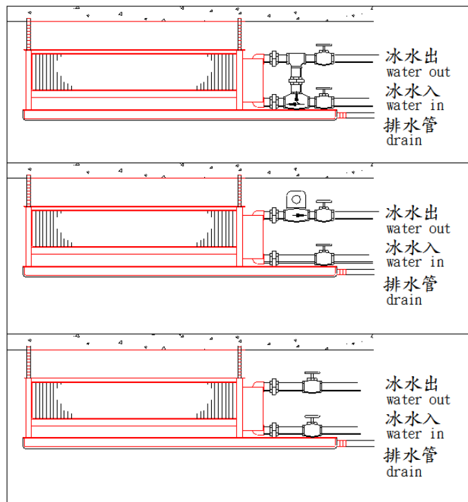
圖(二)水管安裝圖例
